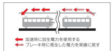
回生ブレーキの仕組み
