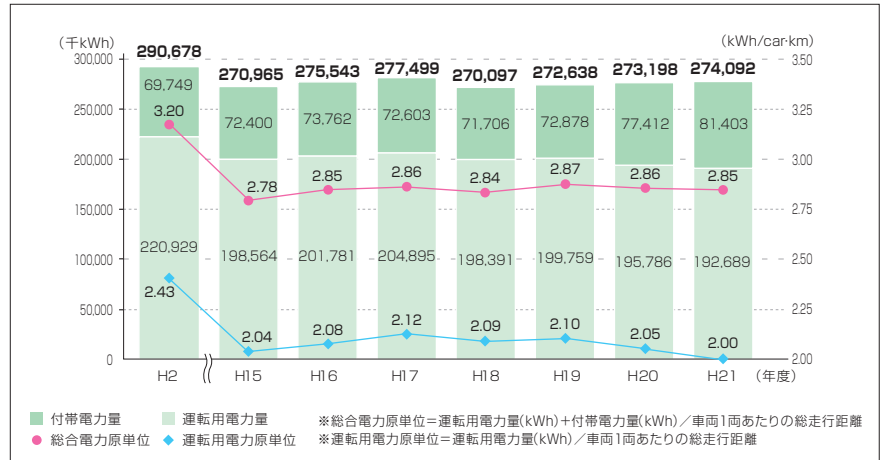
鉄道電力推移
