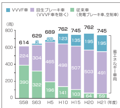
省エネルギー車両の推移
