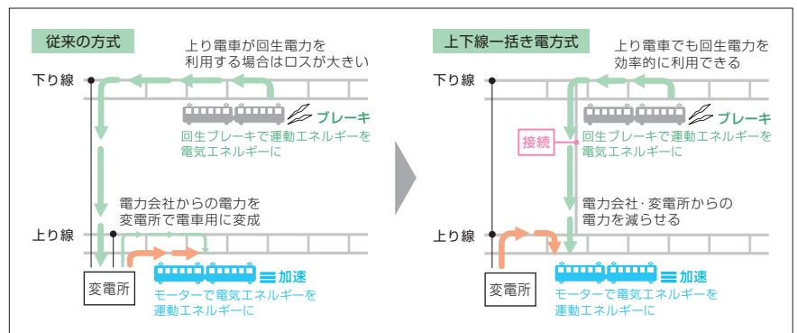
上下線一括電方式の仕組み
